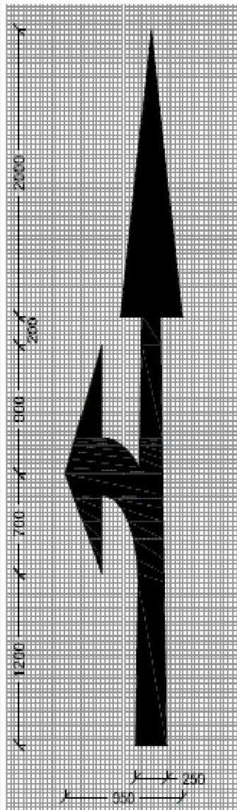
BEA : ευθεία και στροφή αριστερά
