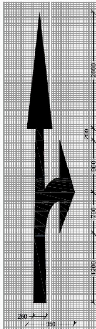
BED : ευθεία και στροφή δεξιά
