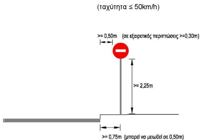
Σχήμα 2. Τοποθέτηση πινακίδων στον ιστό του σηματοδότη
