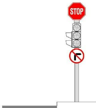
Σχήμα 2. Τοποθέτηση πινακίδων στον ιστό του σηματοδότη
