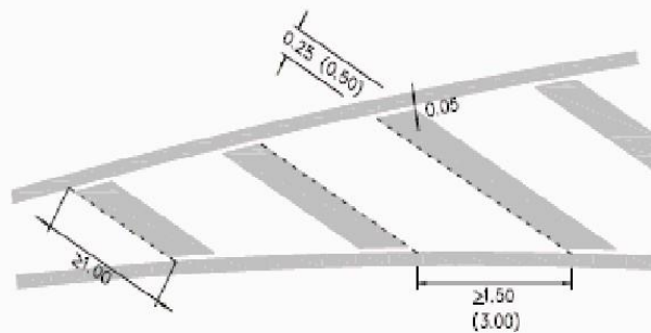
Σχήμα Η2-1: Λεπτομέρεια επιφάνειας αποκλεισμού
