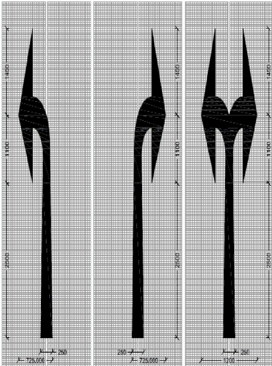
BA : στροφή αριστερά
